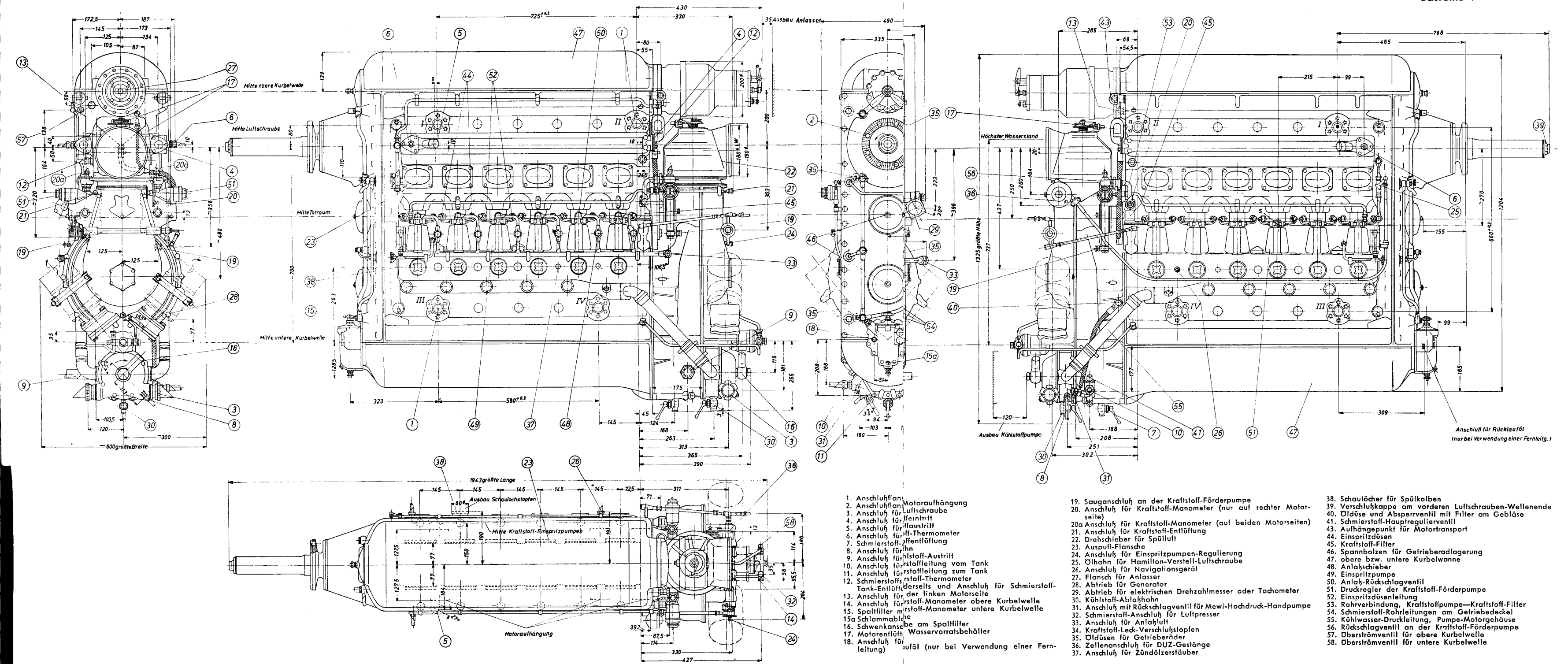
TAFEL 1 Einbauzeichnung JUMO 205 C Baureihe 4
