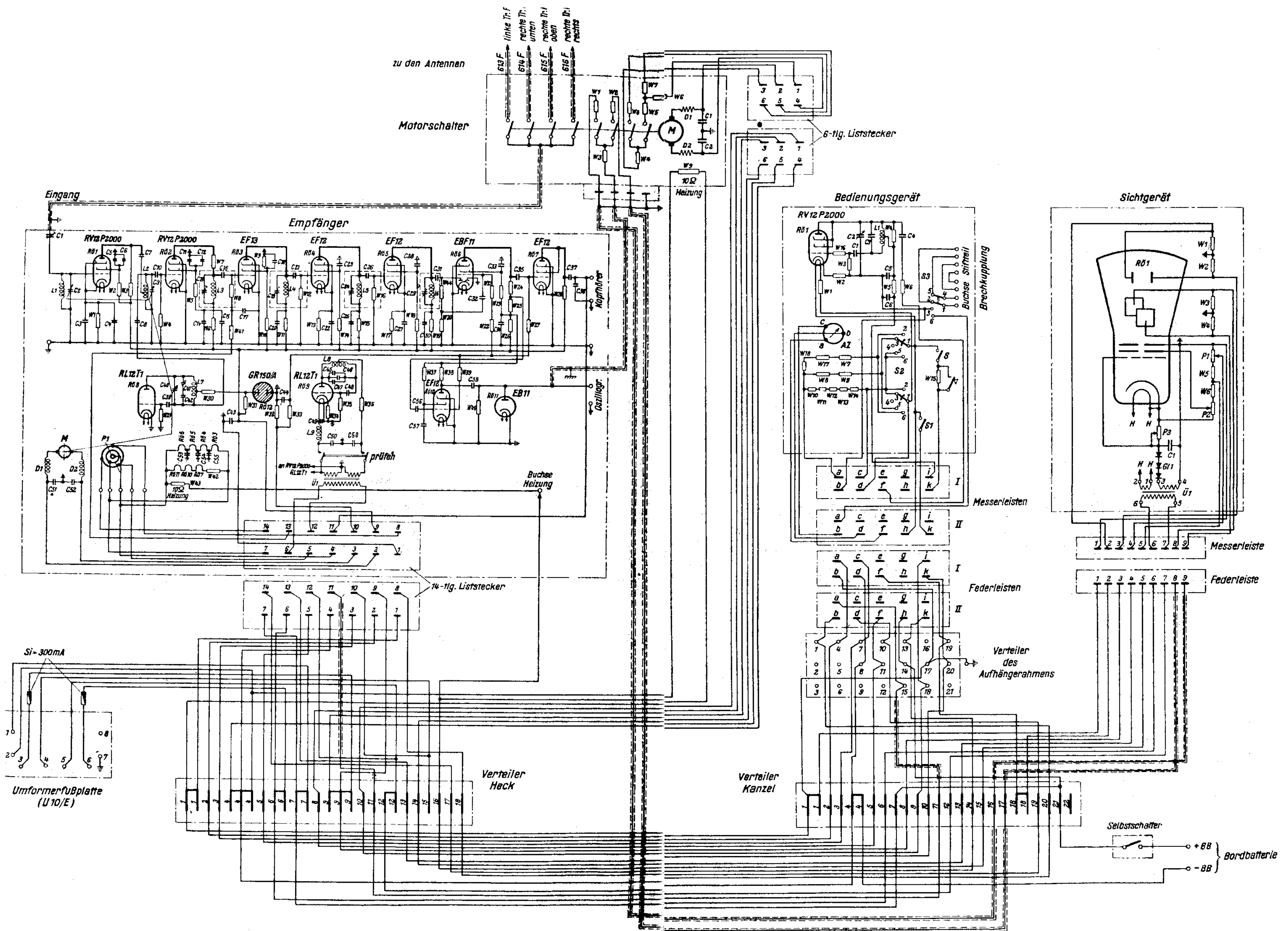
Anl. 1: Gesamtstromlaufplan
