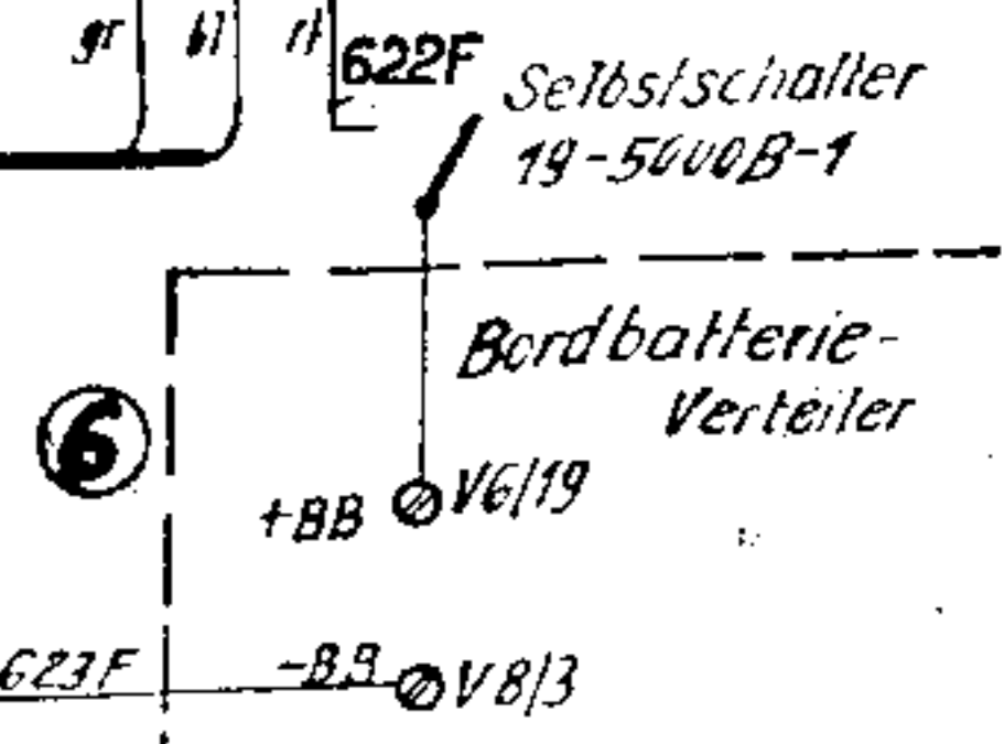
Anl. 2: Prüfschaltplan (alte Ausführung)
