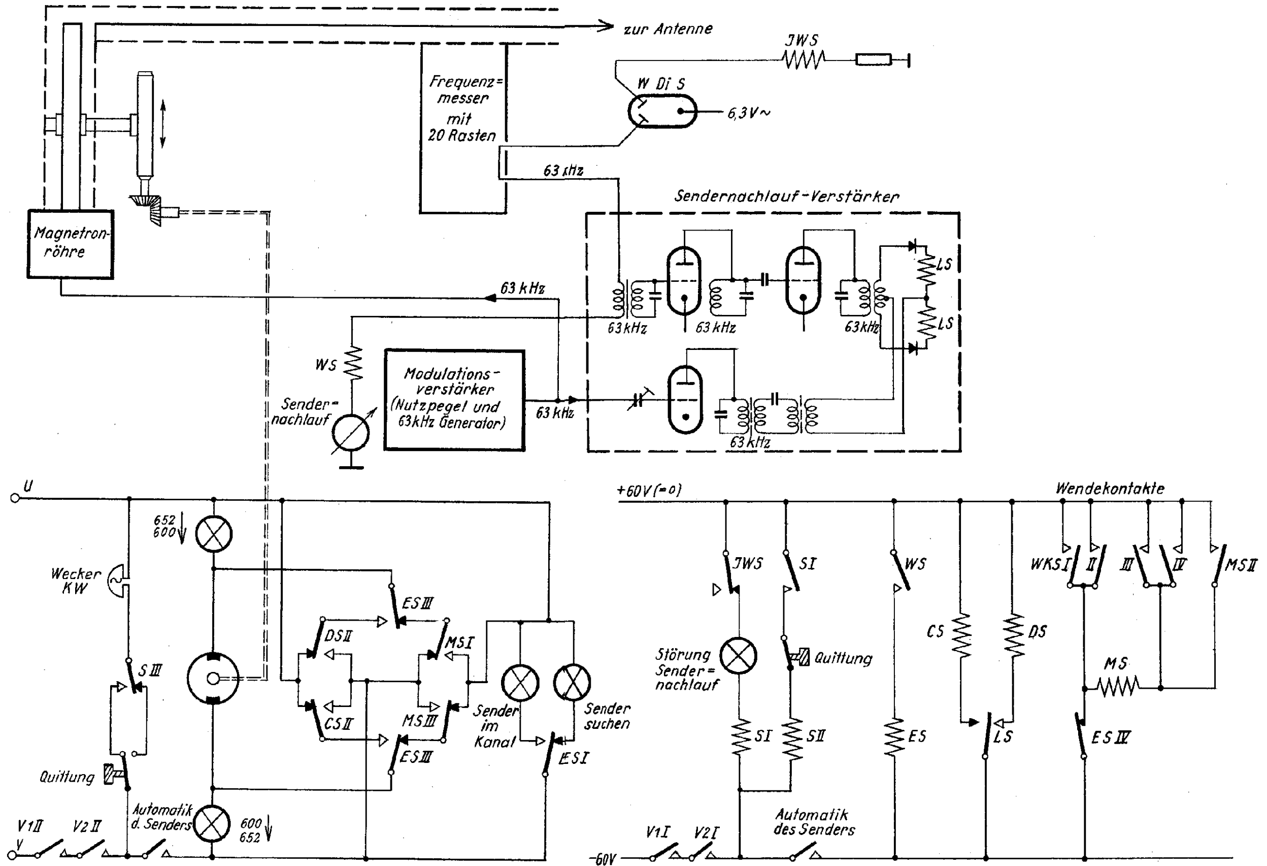
Schaltbild des Sendernachlaufes Anlage 4
